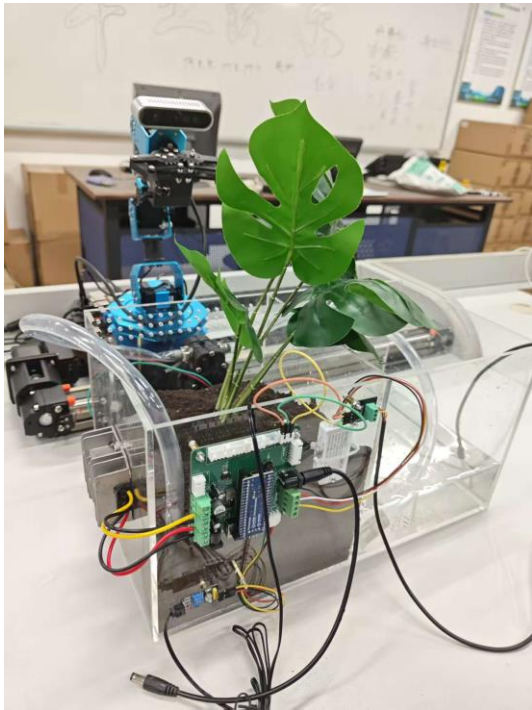
图 1-1 系统实物图
